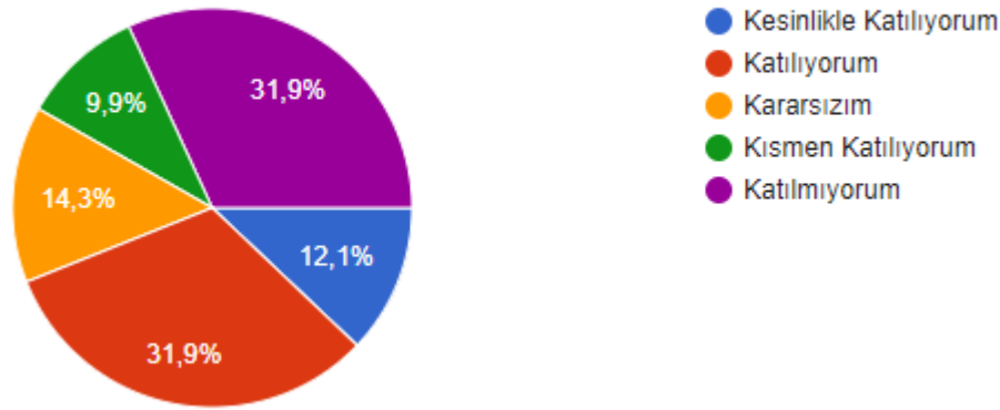
Şekil 3: Velilerin Ulaşılabilirliği
